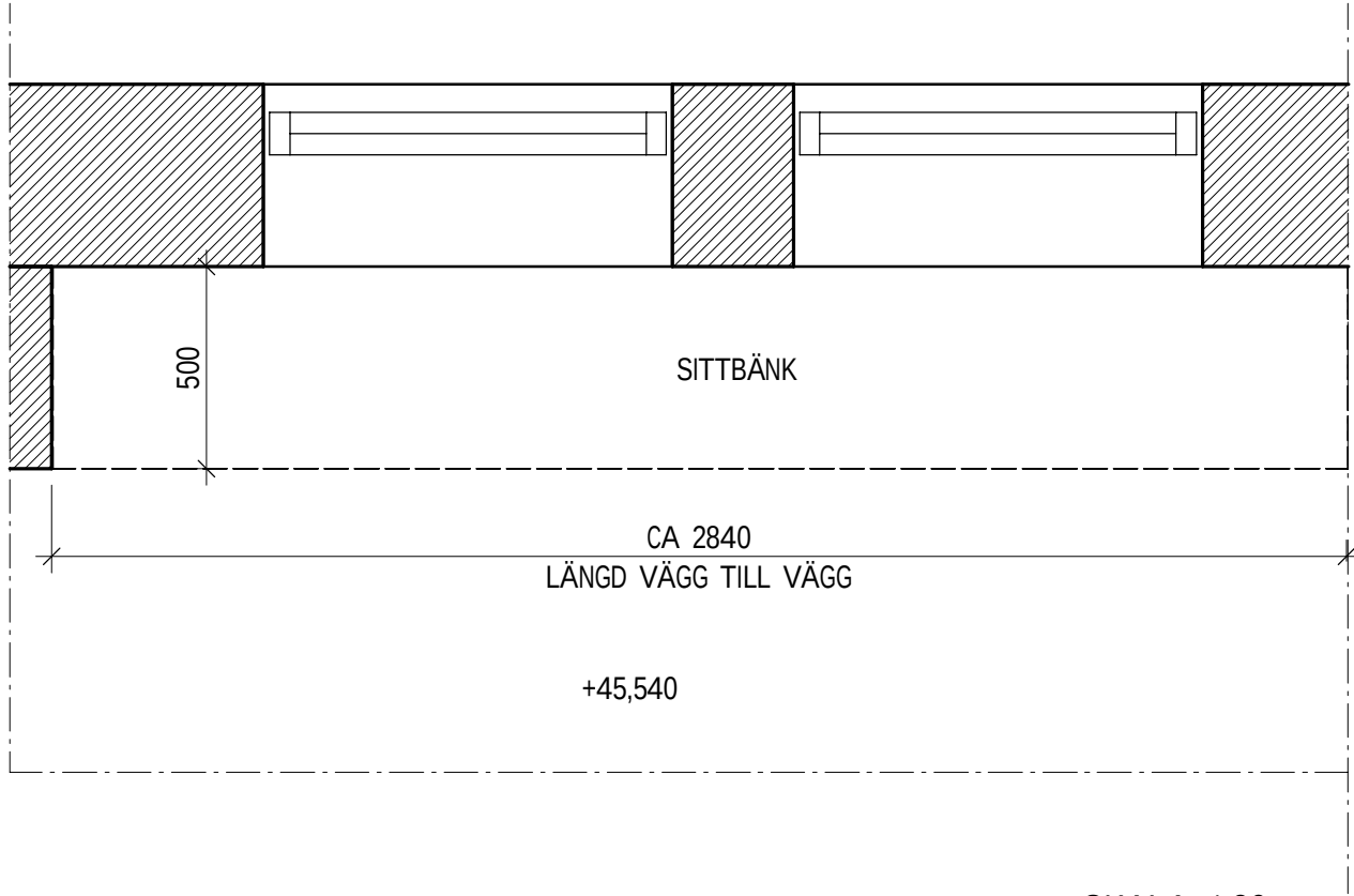
SITTBÄNK I KAPPRUM 1006 - PLAN 1 : 20
