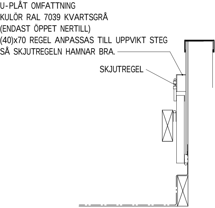
SNITT UPPFÄLLT LÄGE
