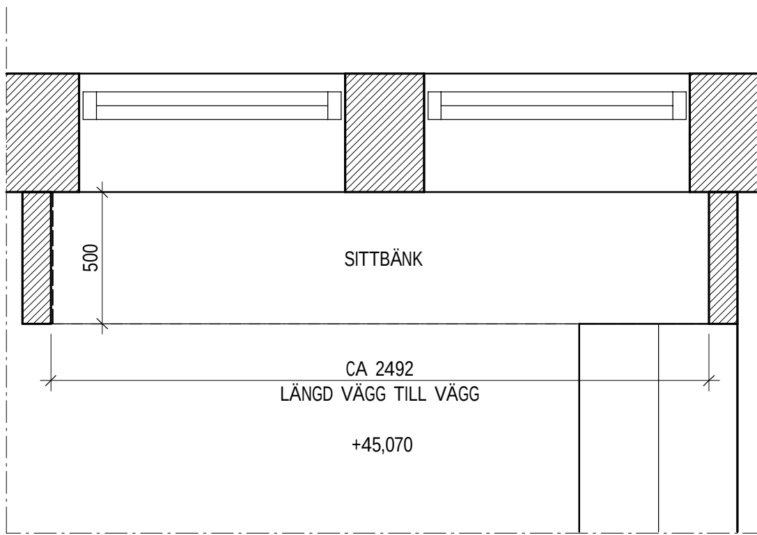
SITTBÄNK I KAPPRUM 1004 - PLAN 1 : 20
