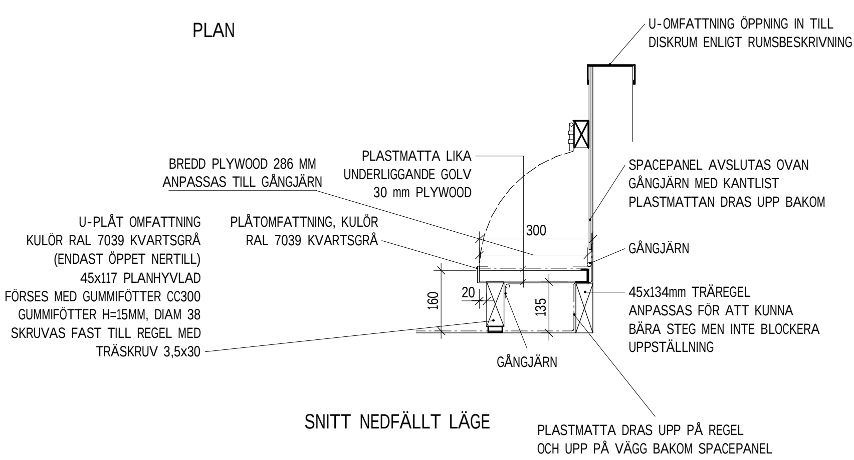
PRINCIPDETALJ STEG I DISKRUM 1 : 10
